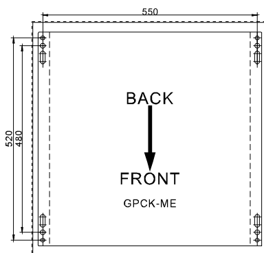
Rys. 6. Szablon montażowy (do użytku w trakcie wiercenia otworów montażowych).
