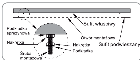
Rys. 8. Montaż ekranu w niskim suficie.
