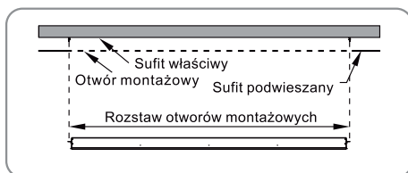
Rys. 6 Użyj śrub do montażu w niskim suficie.
