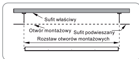
Rys. 7. Użyj szpilek do montażu w wysokim suficie.
