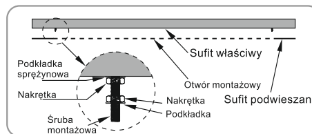
Rys. 8. Montaż ekranu w niskim suficie.
