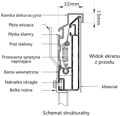
Schemat strukturalny
