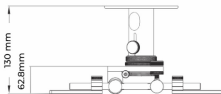
Uchwyt stały
