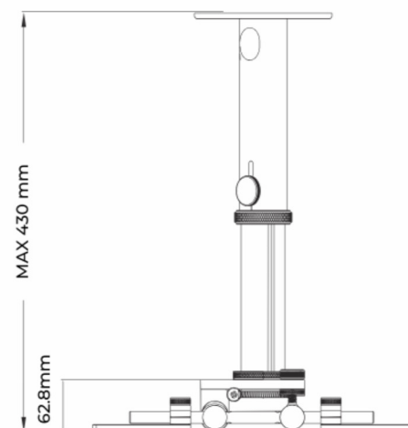
Uchwyt regulowany
